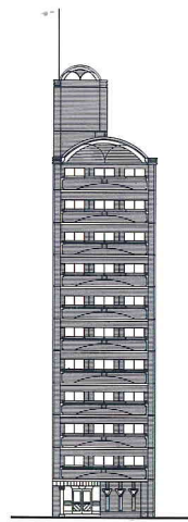
北側立面図
