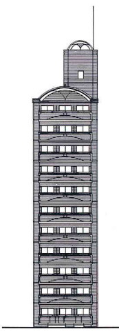
南側立面図
