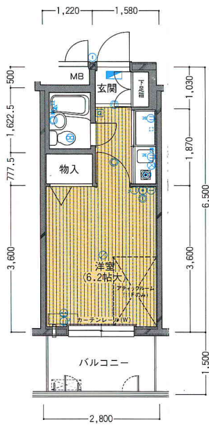
B1TYPE 1ROOM (10戸) ●住居専有面積 18.20㎡ ●バルコニー面積 3.39㎡ ●アタックルーム面積 2.10㎡ (11Fのみ)
