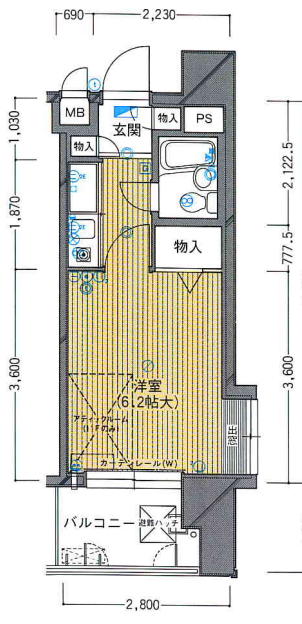
C1TYPE 1ROOM (10戸) ●住居専有面積 18.20㎡ ●バルコニー面積 3.39㎡ ●アタックルーム面積 2.10㎡ (11Fのみ)
