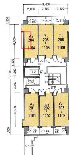
2～11階平面図
